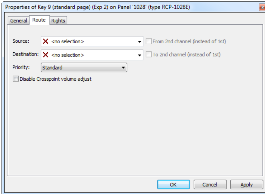
図 569 : Route Audio – Route タブ
