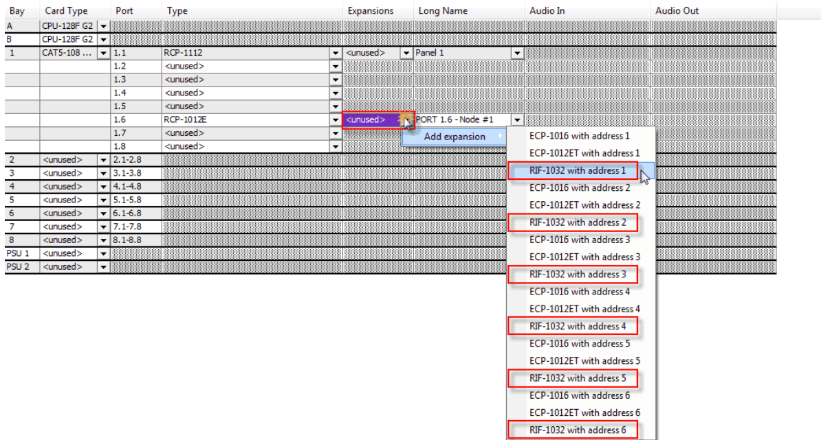
図 669 : RIF - RIF-1032 をエクステンションとして追加する
