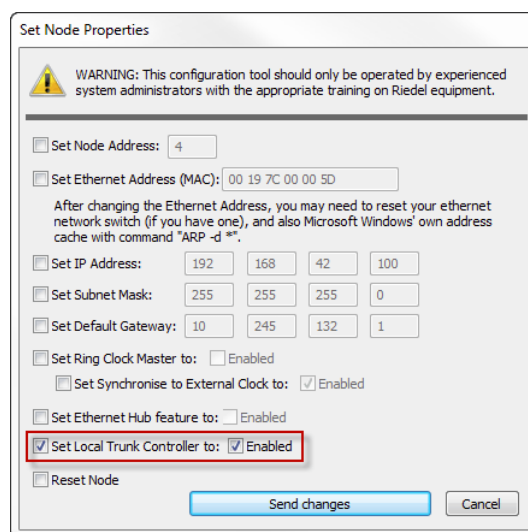
図 869 : Trunking - Director - オンライン・バー - ローカルなトランク・コントローラーを稼動させる
