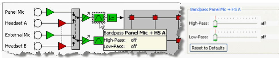
図 147 : Panel Audiopatch - バンドパスのオプション
