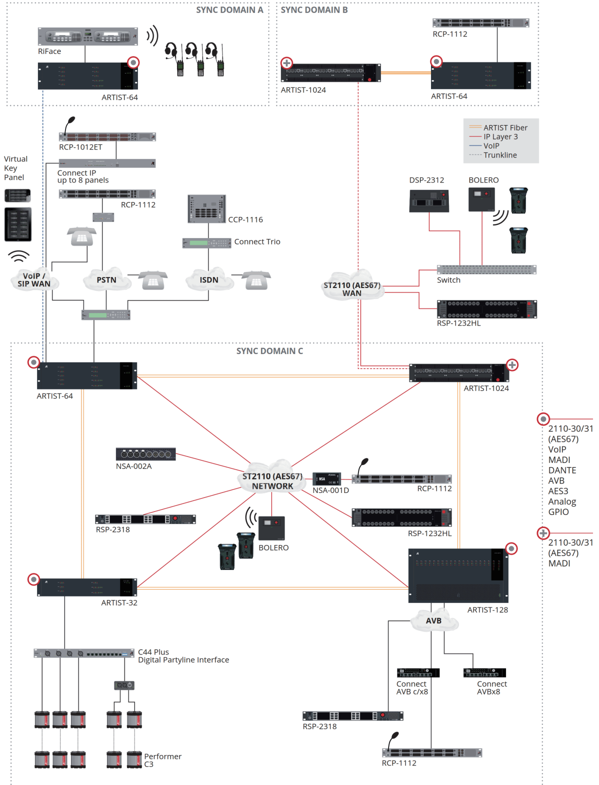
図 3 : Artist システムの設置例
