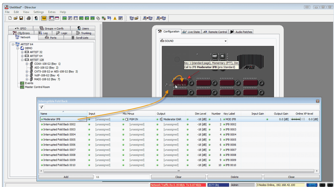
図 177 : IFB-Table – IFB をドラッグ&ドロップする
