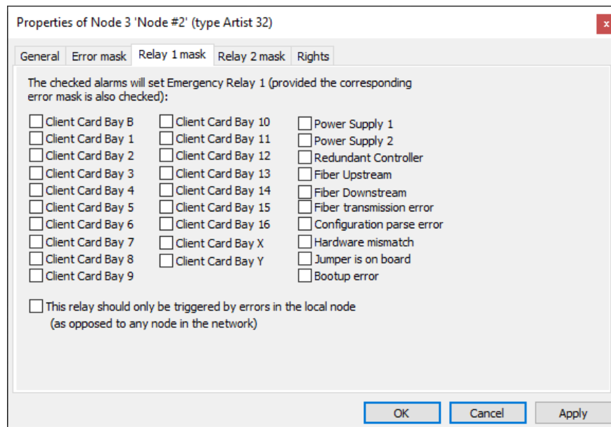
図 384 : ノードのプロパティ - Relay 1 mask タブ
