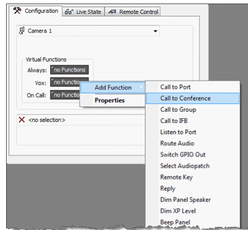
図 199 : Conference - カンファレンスを 4 ワイヤーに割り当てる
