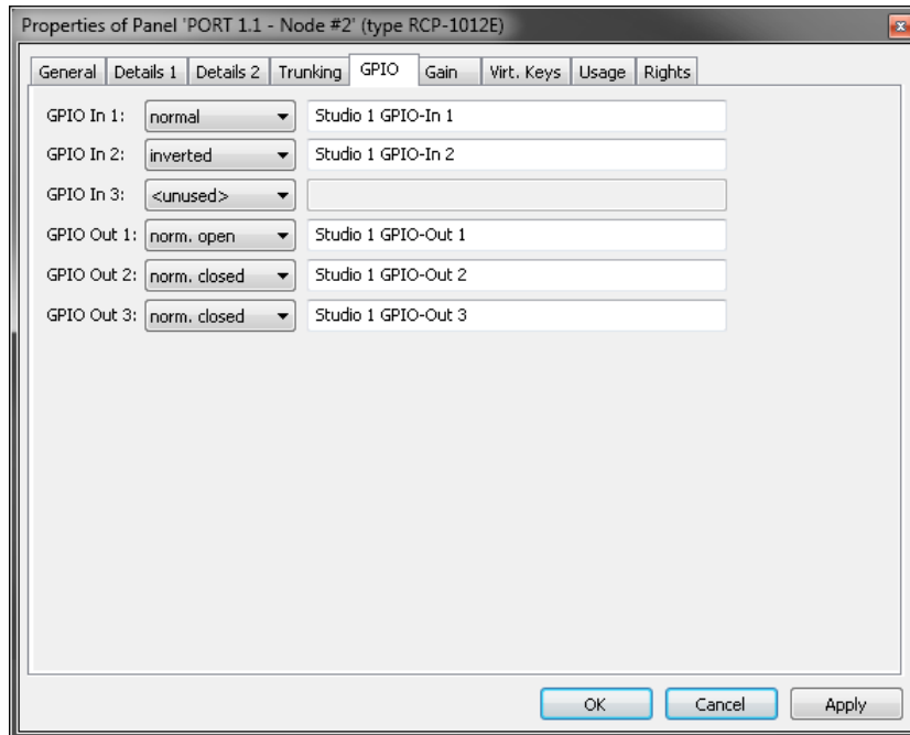
図 414 : パネルのプロパティ - GPIO タブ
