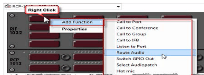
図 680 : RIF - RIF の GPI 入力にコマンドを追加する
