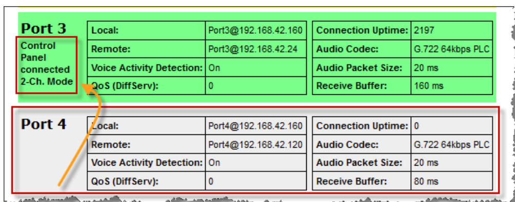
図 481 : CONNECT IPxX - 2チャンネルのパネルのステータス表示
