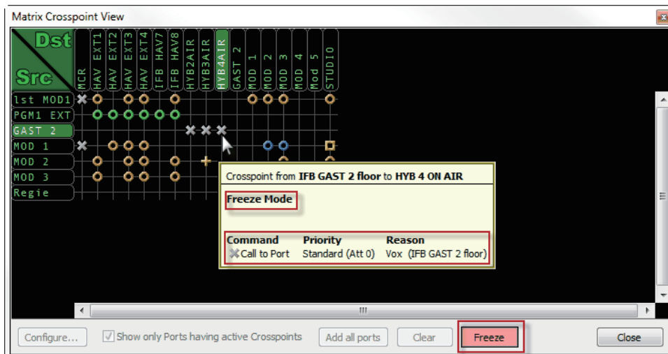
図 288 : Crosspoint View – フリーズ・モード
