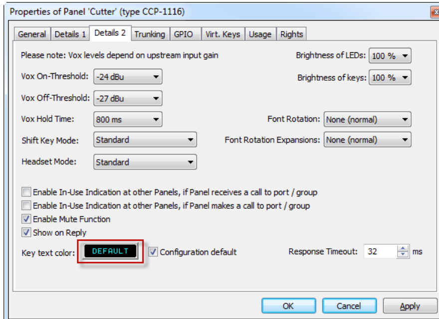
図 532 : 1100/2300 シリーズ - パネルのプロパティ - Details 2 - デフォルトのパネル色を変更する
