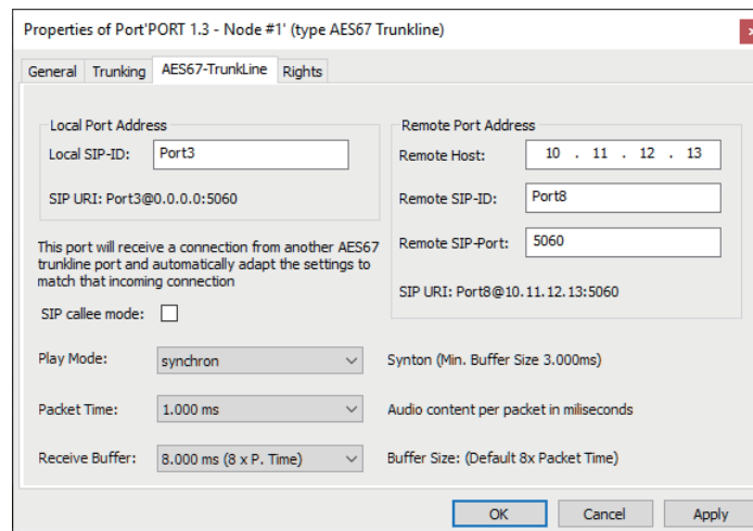
図 427：パネルのプロパティ - AES67 Trunkline タブ
