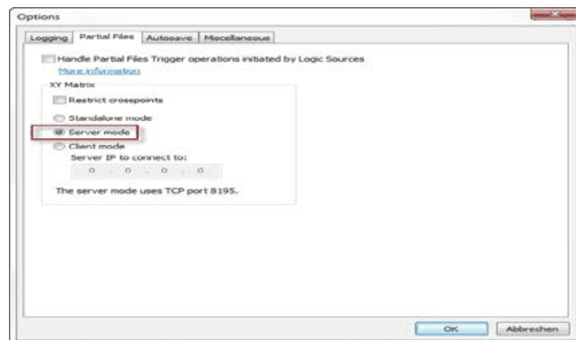
図 706 : Partial File - Options - Server mode のセットアップ
