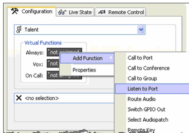
図 160：IFB - リッスン・ソースを追加する
