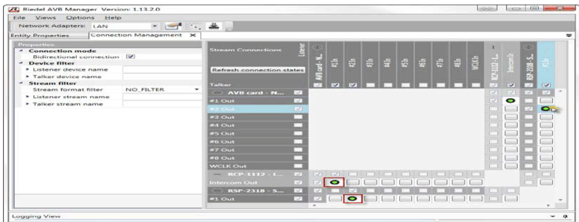
図 524 : AVB-Manager – クロスポイントを作成する
