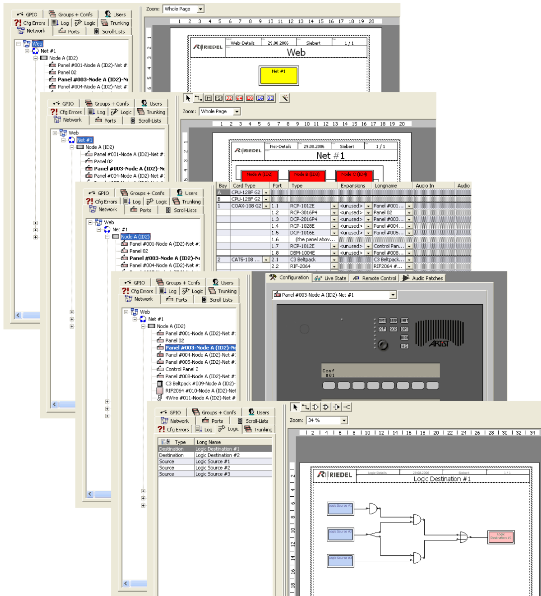
図 358 : Director - ナビゲーション・バー - ワークスペース
