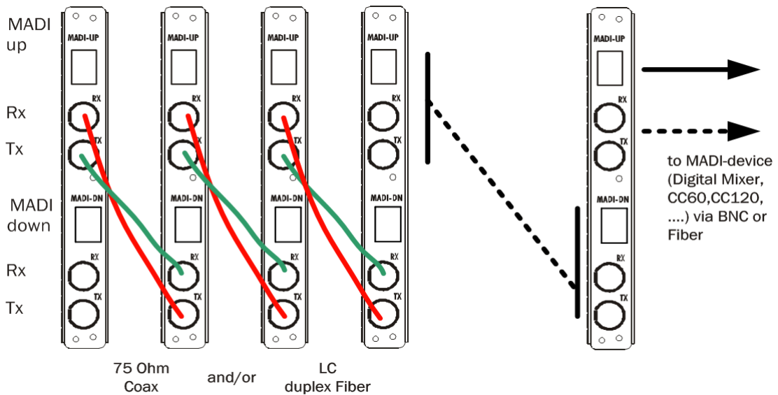
図 431 : MADI-カードをカスケード接続する
