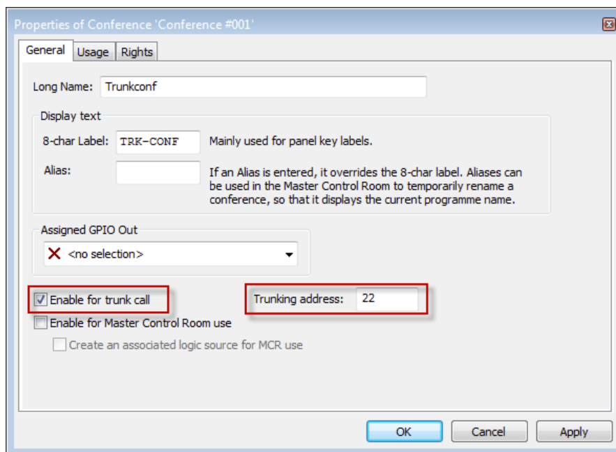
図 926 : Trunking – Call to Group/Conference – トランキング・アドレス
