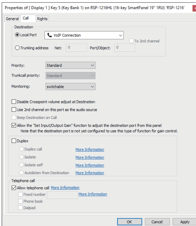
図 563 : Call to port – Call タブ
