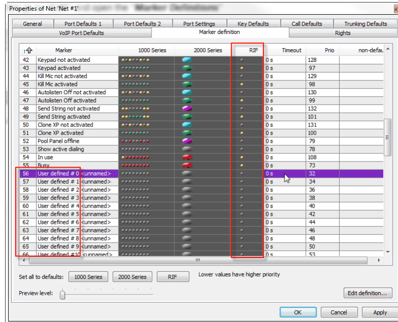
図 674 : RIF - Marker Definitions - ユーザー定義の RIF
