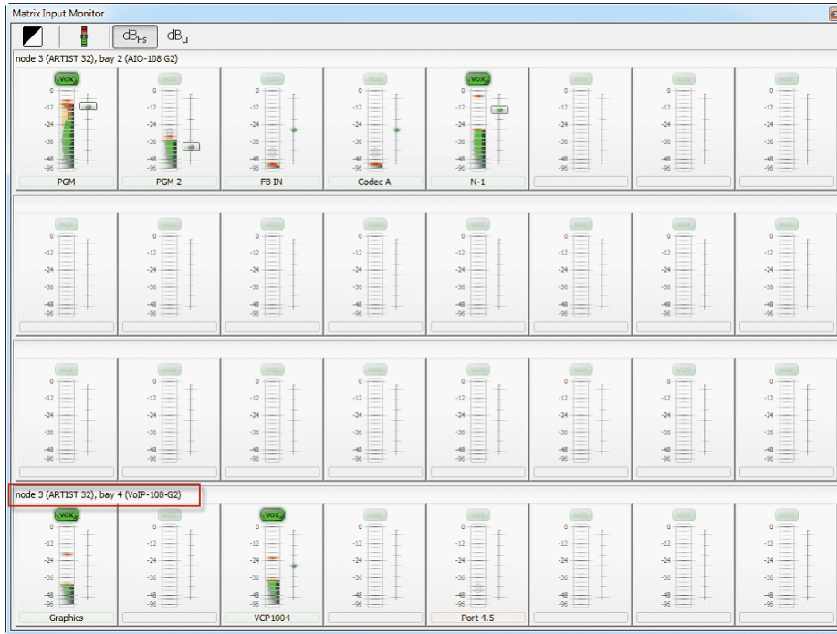
図 297 : Matrix Input Monitor – 新クライアント・カードの表示
