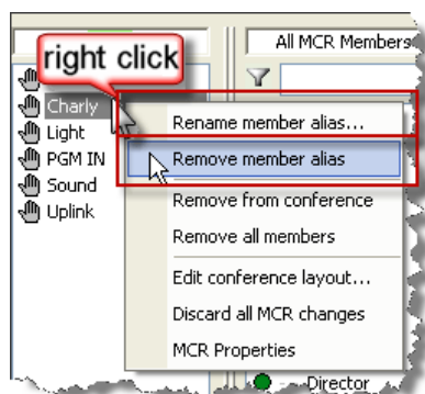
図 771 : MCR の使用法 - エイリアスの名前を変更するまたはエイリアスを削除する
