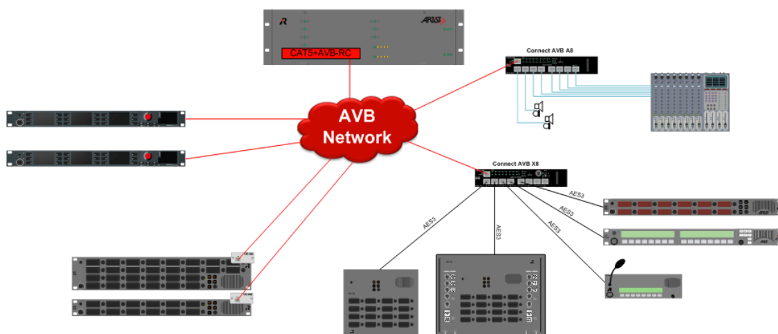
図 516 : Artist AVB ネットワーク
