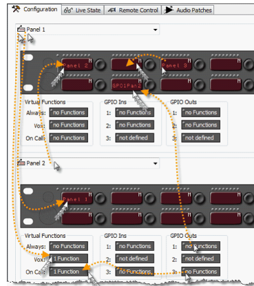
図 128 : Add function - デスティネーション・パネル上のキー割り当て
