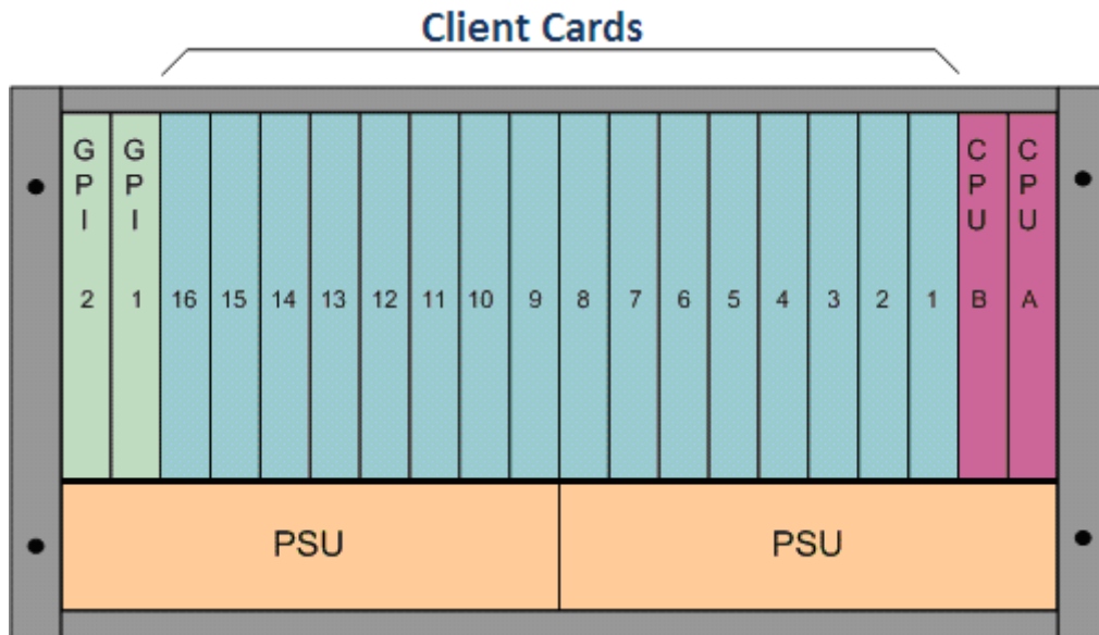
図 49 : Artist-M/128 のベイの番号付け, 正面図
