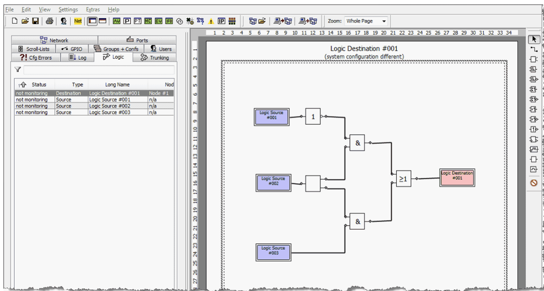
図 242 : Logic - ロジック・ワークスペース
