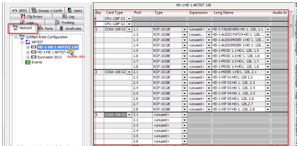
図 83 : ノードのコンフィギュレーション : ポートを移動する - 希望するノードの Node Configuration ビュー
