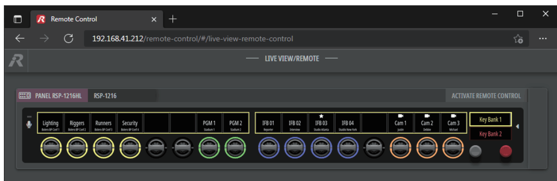
図 273 : パネルのライブ・ステート - ライブ・ステートのモニタリング (Artist-1024)
