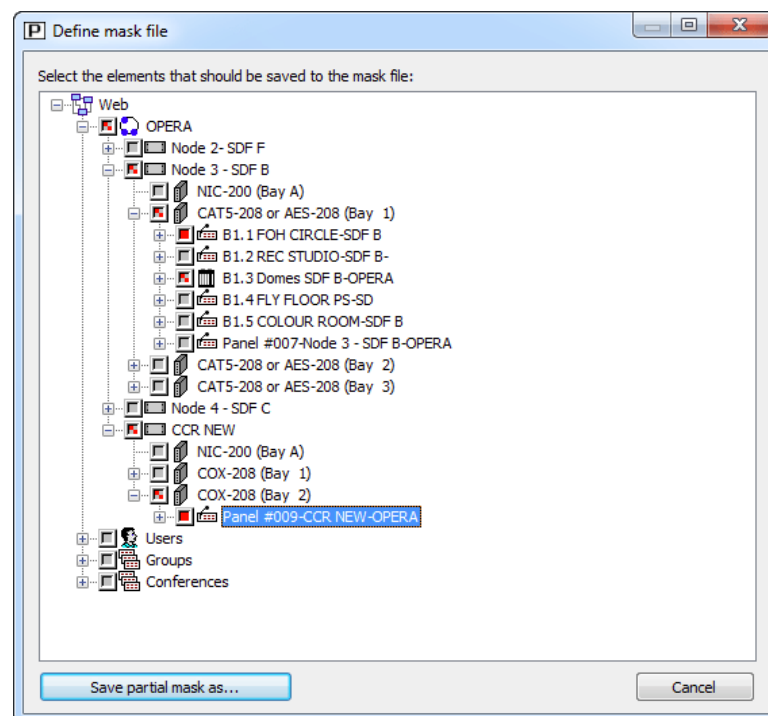
図 687 : Partial Files – マスク・ファイルを定義する
