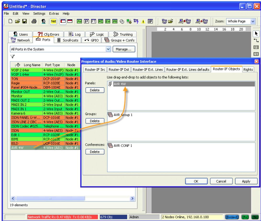
図 856 : AV Router - 4 ワイヤーを追加する
