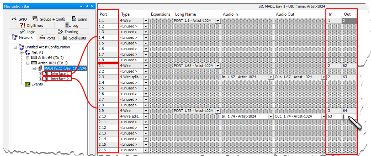
図 437 : Artist-1024 - 個別 MADI ポートをマッピングする
