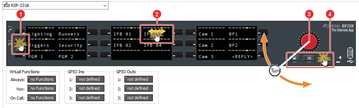
図 269 : 2300 シリーズ SmartPanel のリモート・コントロール (Artist-32/64/128)
