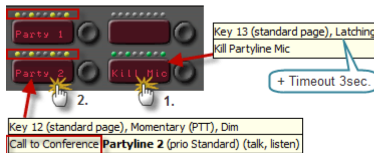
図 592 : Kill Partyline Mic – パネルの操作
