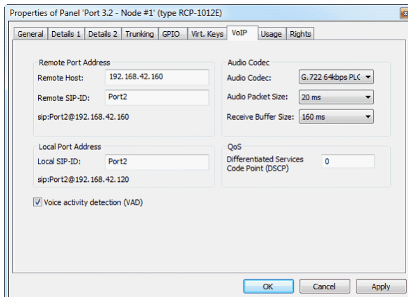
図 468 : VoIP - VoIP ポートのプロパティ
