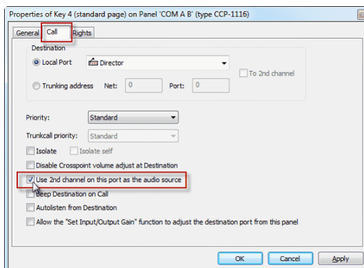
図 656 : CCP 1116 - コメンテーター B の機能用の第 2 音声チャンネル
