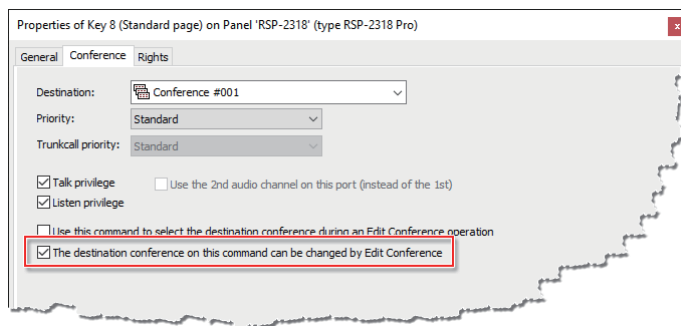
図 205 : Edit Conf - このコマンド上のデスティネーション・カンファレンス...
