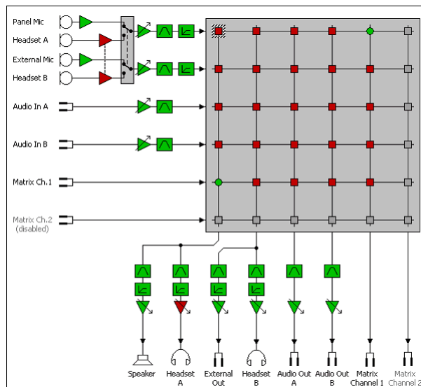
図 115 : パネルのオーディオ・パッチ
