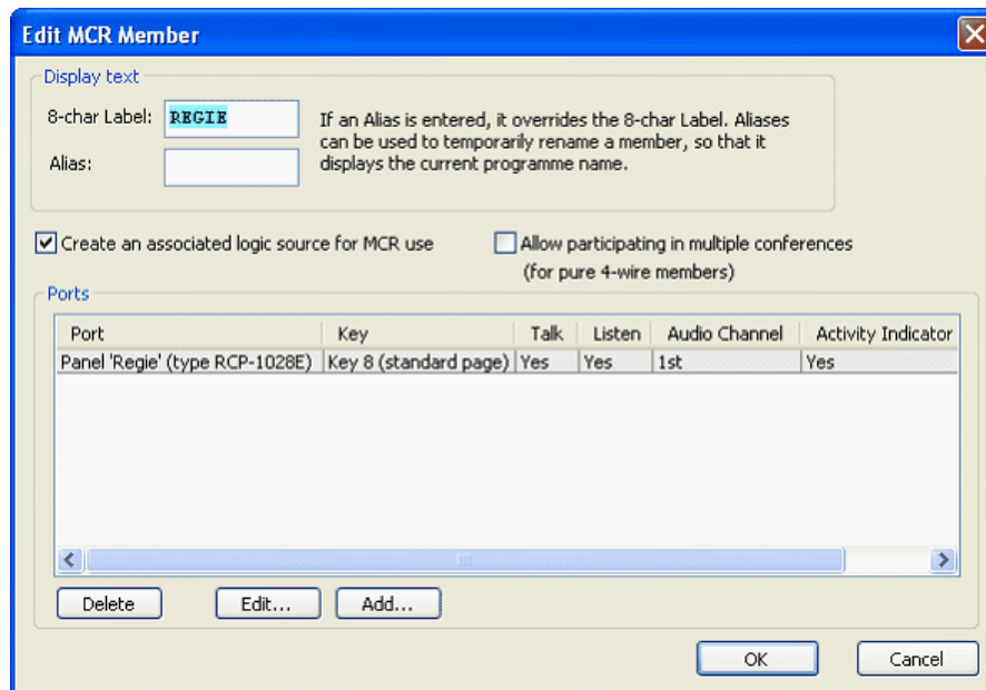
図 728 : MCR - MCR のメンバーを編集する
