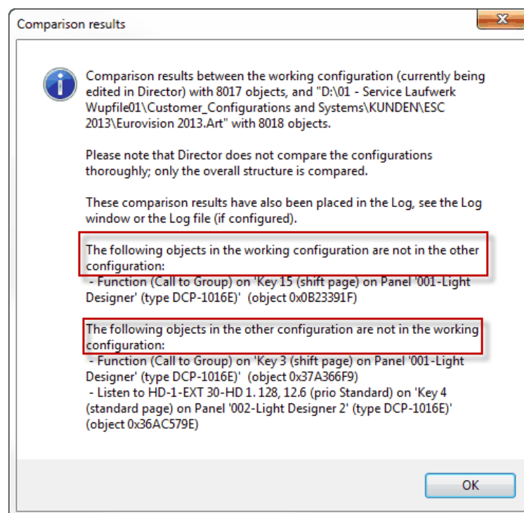
図 323 : File - Compare with... : 比較結果のウィンドウ
