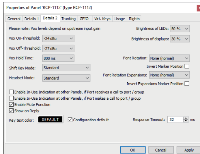
図 402 : ポート / パネルのプロパティ - Details 2 タブ
