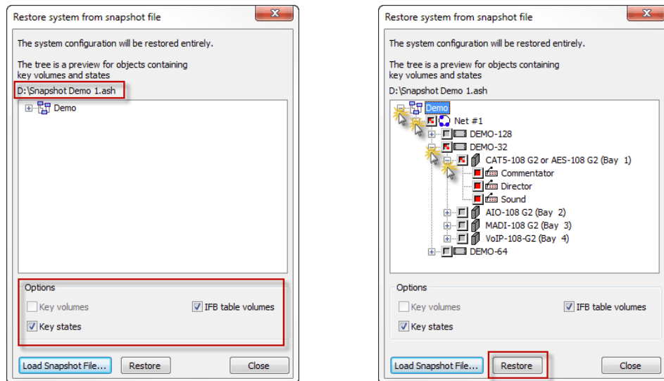
図 101 : リストアする要素
