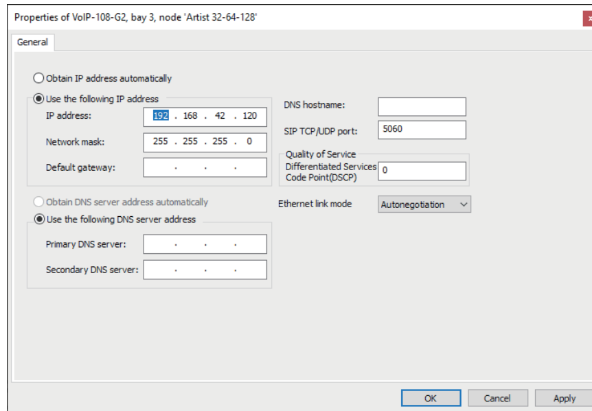
図 397 : VoIP カードのプロパティ - General タブ
