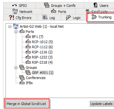
図 227 : トランキング - ナビゲーション・バー
