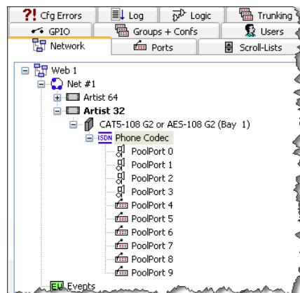
図 634 : Connect - ネットワーク・ビュー内のプール・パネル
