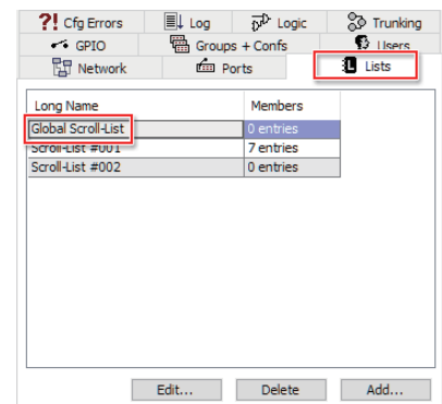
図 226：グローバル・スクロール・リスト—ナビゲーション・バー
