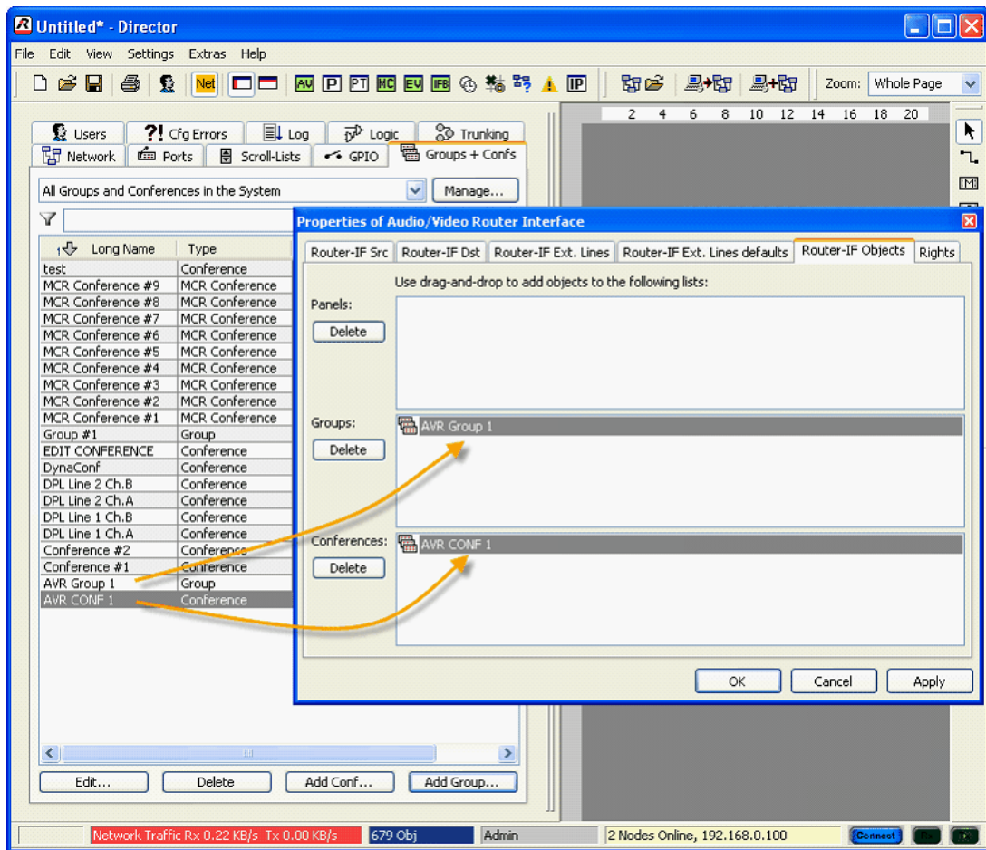
図 848 : AV Router - グループとカンファレンスを AVR に追加する
