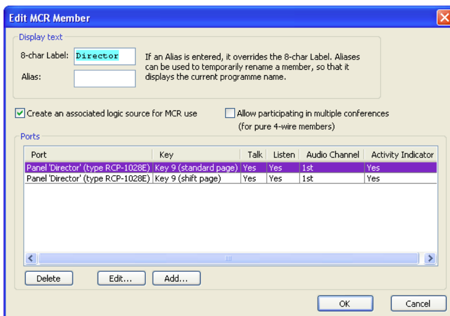
図 731 : MCR - 新規 MCR メンバーを追加する - 例
