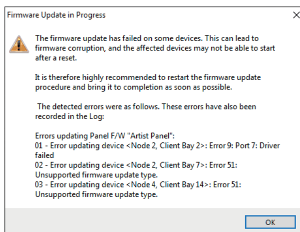
図 315 : Firmware Update – Panel – 非互換パネルのエラー・メッセージ
