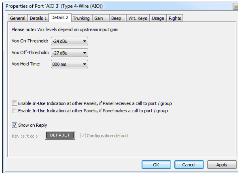
図 551 : 4 ワイヤーのプロパティ - Details 2 タブ
