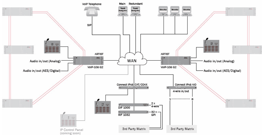
図 470 : CONNECT IPx2/x8 - 使用例
