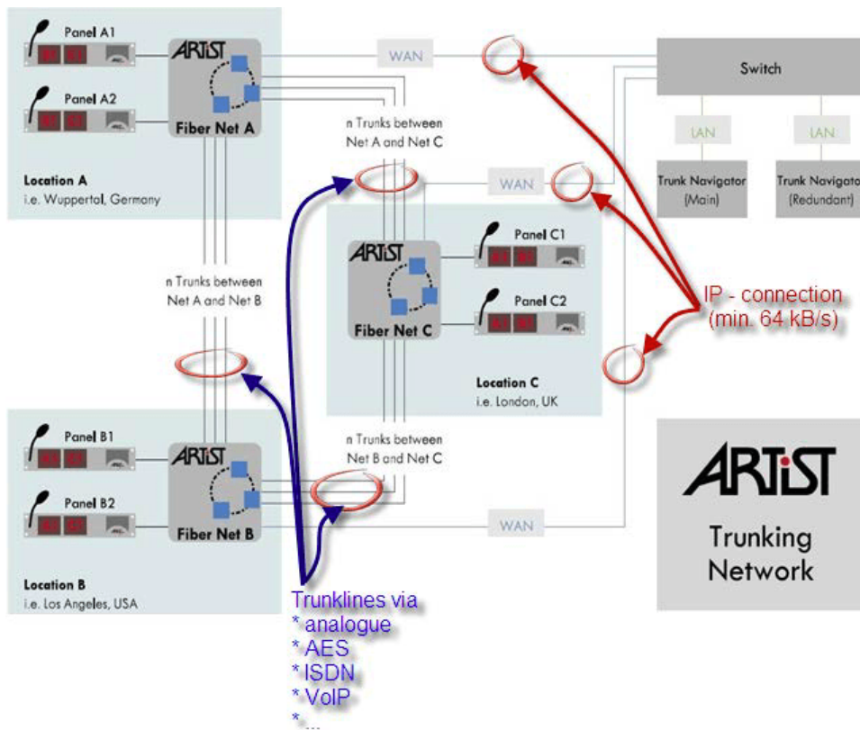
図 867 : Trunking – トランク接続されたネットワークを構築する
