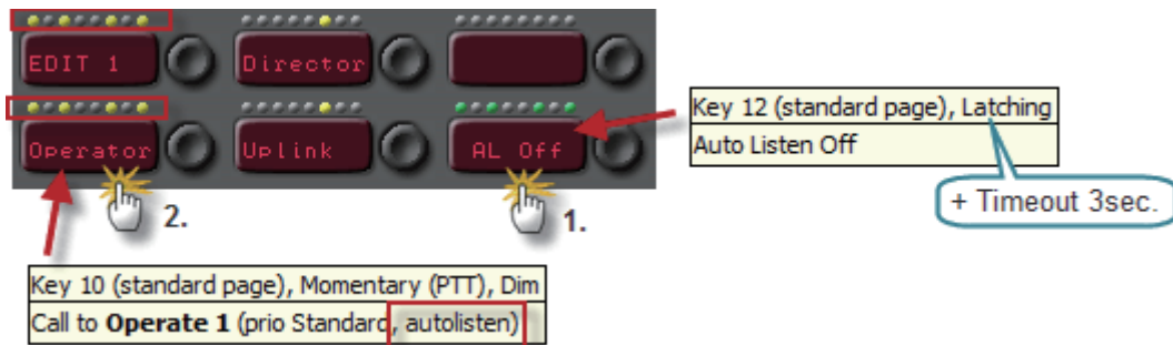
図 594 : Autolisten Off – パネルの操作
