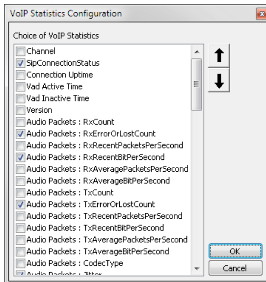
図 514 : VoIP statistics コンフィギュレーション
