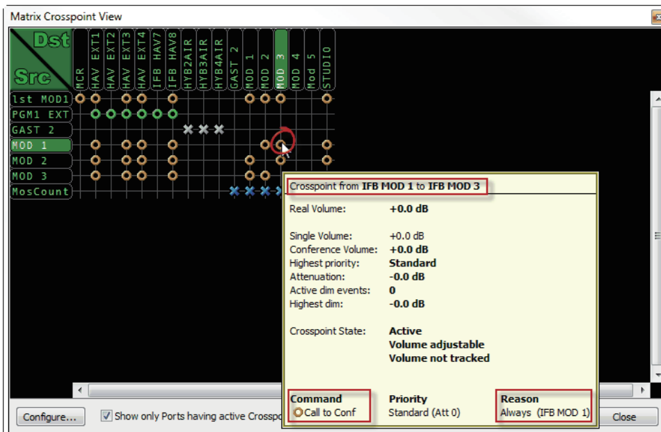
図 285: クロスポイント・ビュー-クロスポイントの情報
