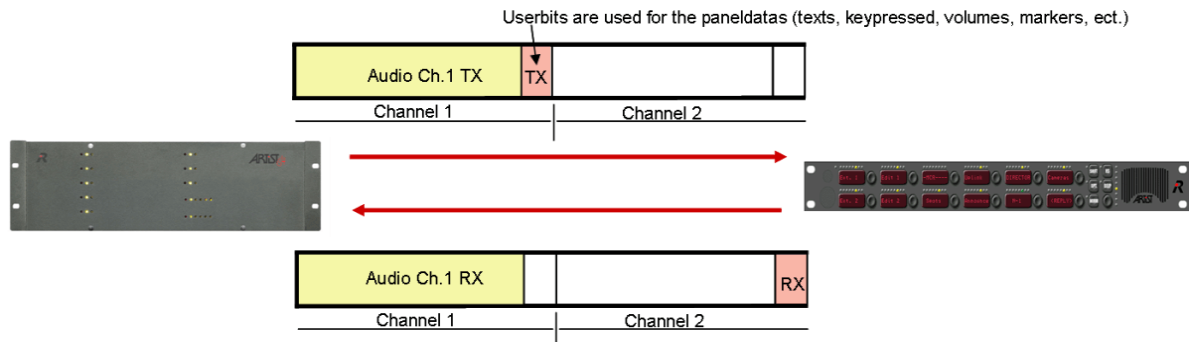
図 78 : Artist とパネルの間の 1 つの AES チャンネルを用いた通信
