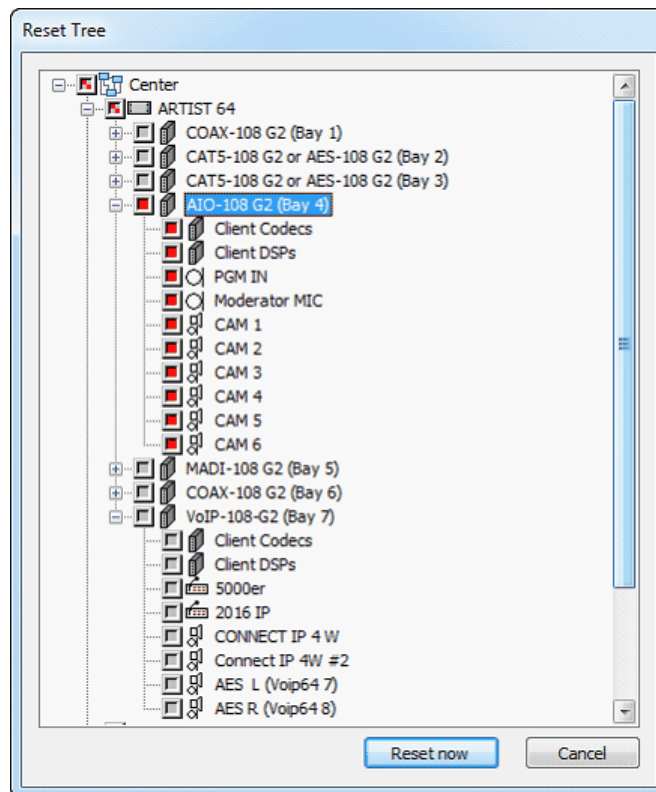
図 343 : メニュー・バー - Extras - Reset Tree...
