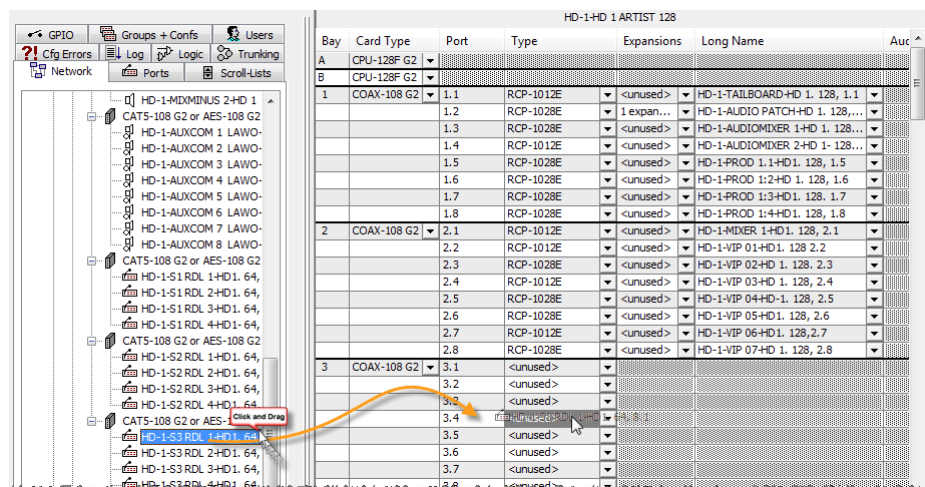
図 84 : ノードのコンフィギュレーション : ポートを移動する - ポートをドラッグ&ドロップで移動する
