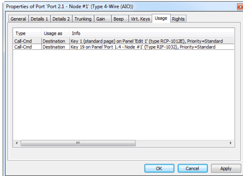
図 557 : 4 ワイヤーのプロパティ - Usage タブ
