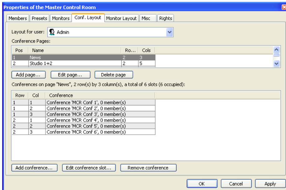
図 739 : MCR - レイアウト - MCR のプロパティ
