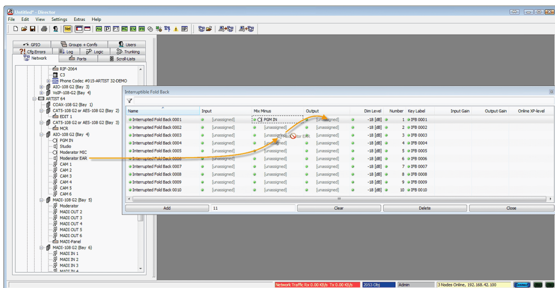
図 174 : IFB-Table - ドラッグ & ドロップによる割り当て
