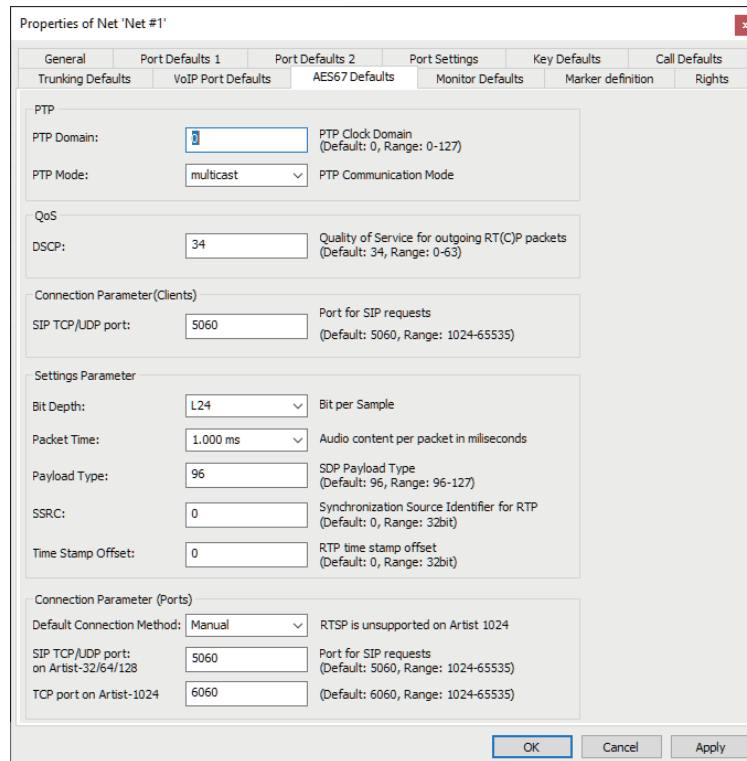
図 375 : ネットのプロパティ - AES67 Defaults タブ
