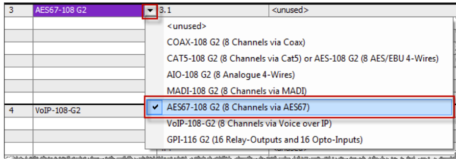
図 440 : AES67 カードをノードのコンフィギュレーションに追加する
