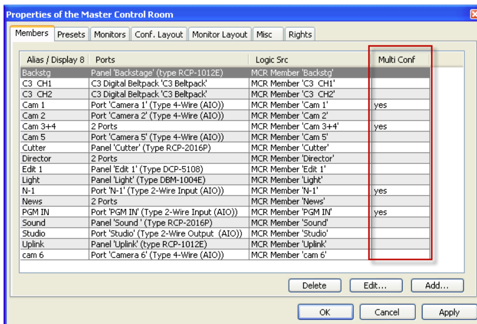
図 734 : MCR - メンバー - テーブル - Multiconf
