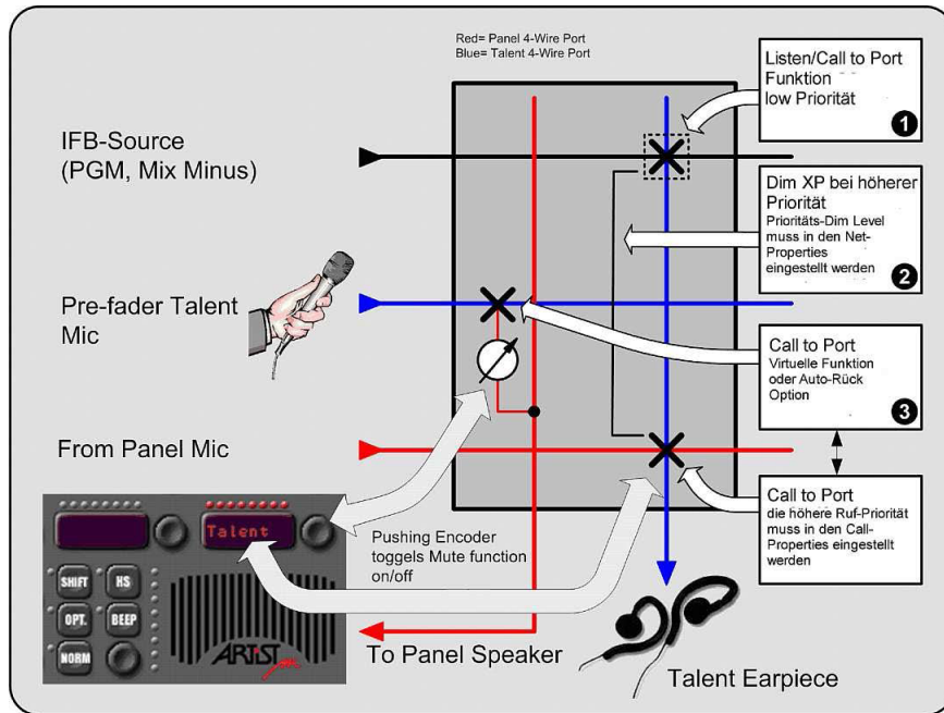
図 164：IFB - プロパティを使って IFB を設定する
