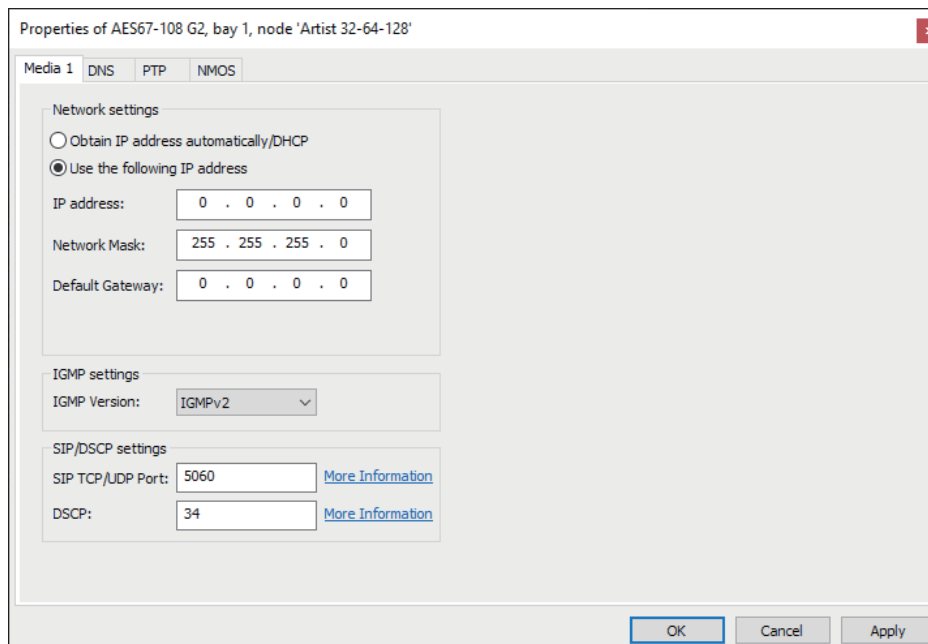
図 442 : AES67-108 G2 カードのプロパティ
