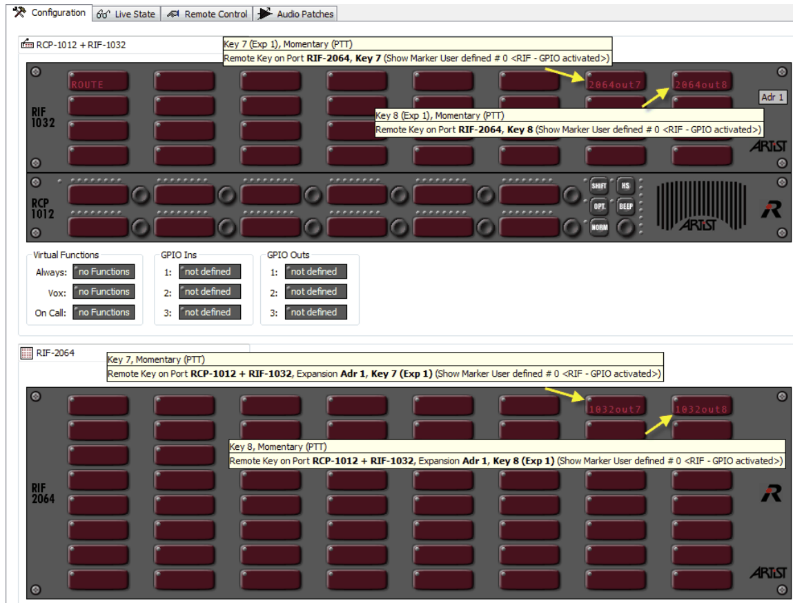
図 683 : RIF - RIF から RIF へのコンフィギュレーション例
