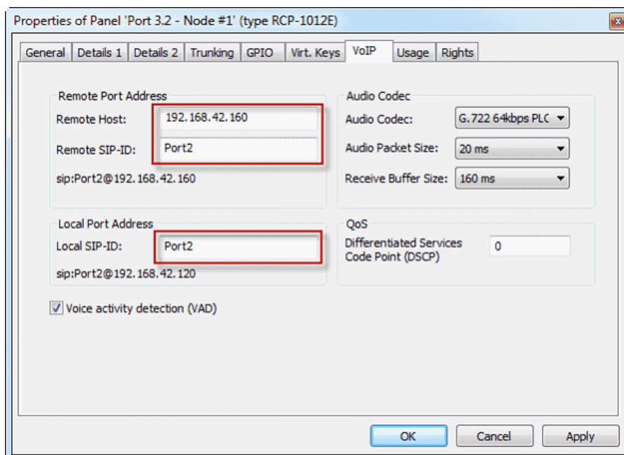
図 483 : CONNECT IPxX - Director - ポートのコンフィギュレーション
