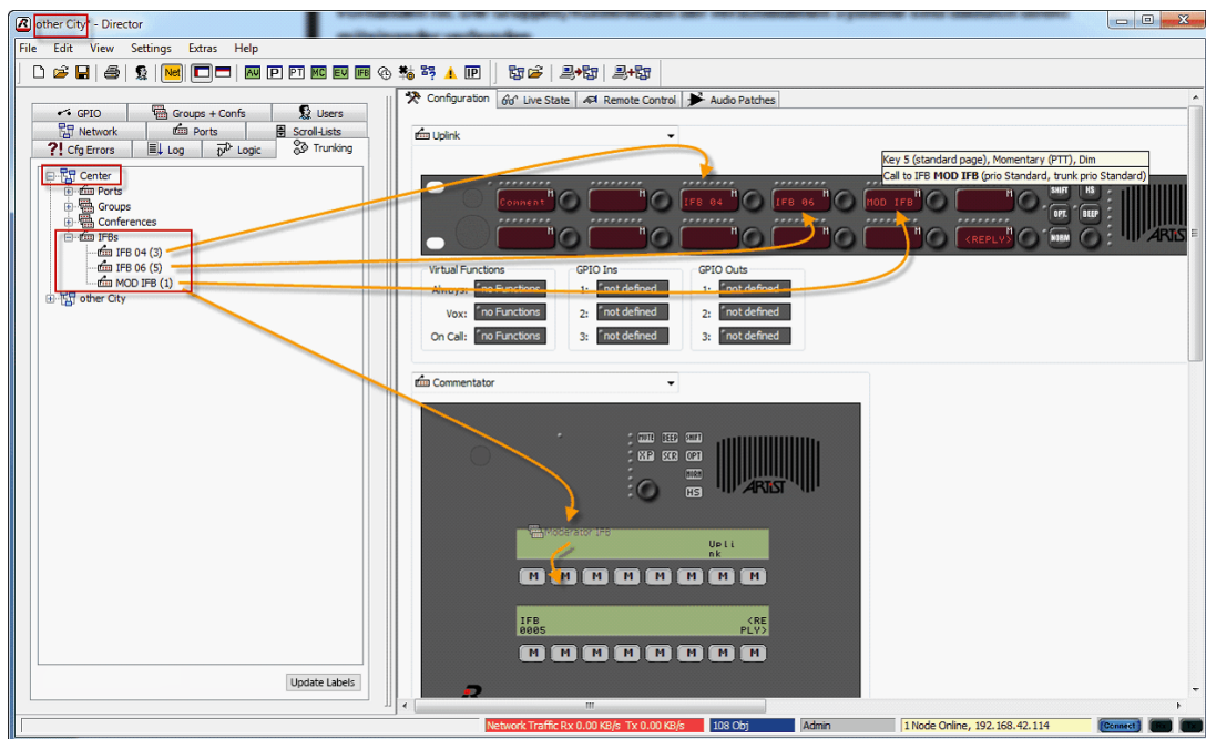
図 928 : Trunking - 「Call to IFB」を設定する
