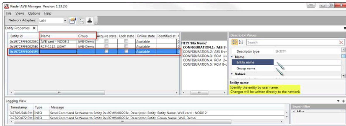
図 521 : AVB-Manager – 名前とグループ・ラベル
