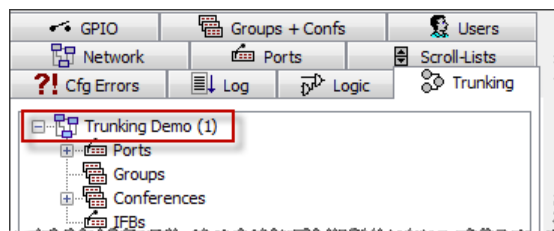
図 873 : Trunking - ネット・ラベルとアドレスを表示する Trunking タブ
