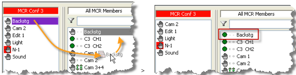
図 765 : MCR の使用法 - メンバーをカンファレンスから削除する
