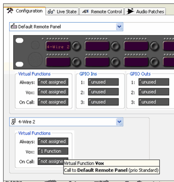
図 134 : 4ワイヤー用の Auto Reverse Talk の例
